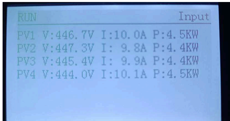
Figura 08 – Tela do inversor nº3 - Foz do Iguaçu
