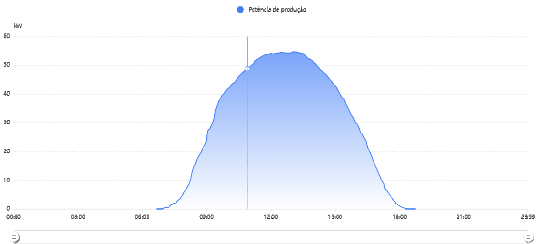
Figura 07 – Gráfico de geração (aplicativo Solarman) - Foz do Iguaçu
