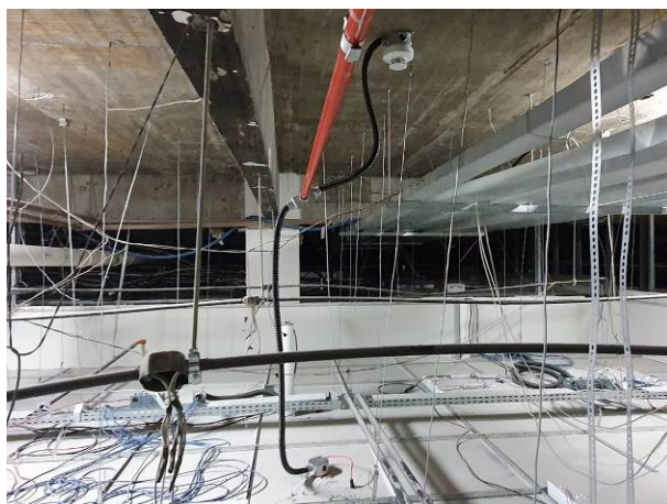
Figura 07: Infraestrutura, detector de fumaça acima do forro e sinalizador de acionamento
