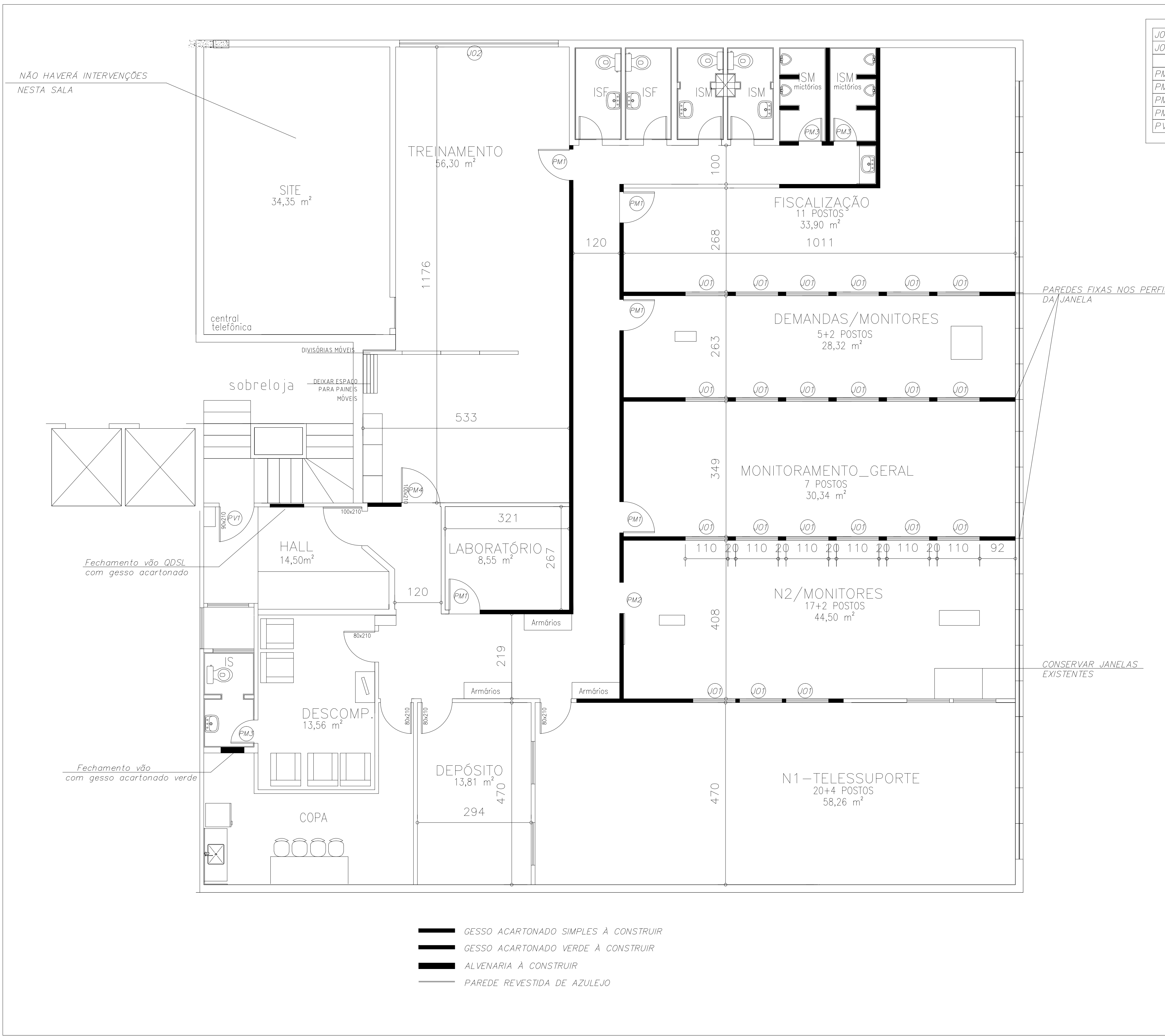
PLANTA CONSTRUÇÃO - SOBRELOJA Escala 1:50
